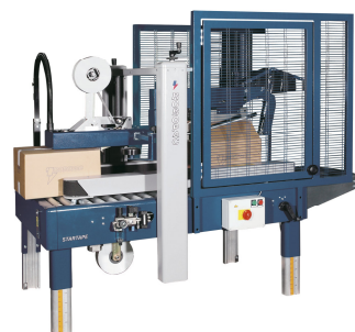
Fermeuse de caisses automatique Scotcheuse mono-format Grande cadence sans opérateur Fermeture des rabats automatiques
