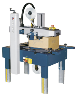
Fermeuse de caisses mono-format Entrainement supérieur / inférieur Ou entrainement latéral Réglage manuel
