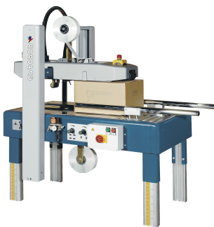
Fermeuse de caisses multi-format Scotcheuse multiples dimensions 2 formes d'entraînement possible Réglage automatique
